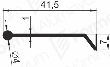
Pr.No: 8590 0,14 kg/m
