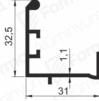
Pr.No: 8591 0,300 kg/m
