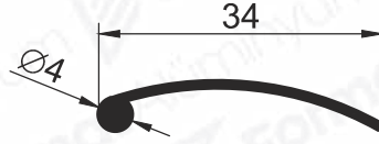
Pr.No: 9111 0,104 kg/m
