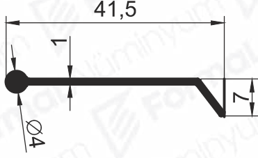
Pr.No: 8590 0,147 kg/m
